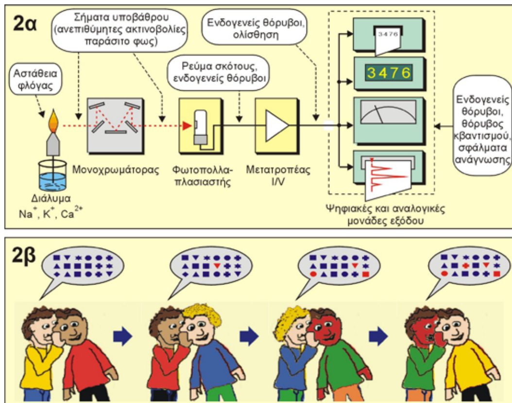
Σχήμα 2: (α) Σχηματική παράσταση μιας φλογομετρικής διάταξης, όπου η πληροφορία (ένταση εκπομπής ατομικής ακτινοβολίας του μετρούμενου στοιχείου) διέρχεται από μια αλληλουχία επιμέρους οπτικών και ηλεκτρονικών μονάδων, καθεμία των οποίων προσθέτει διάφορους τύπους θορύβου, που όλοι μαζί συμβάλλουν σε μια συνολική αλλοίωση της ζητούμενης πληροφορίας. (β) Το «ανάλογο» είναι το γνωστό «σπασμένο τηλέφωνο»: Ένα άτομο μεταφέρει μια πληροφορία σε ένα άλλο, το άλλο σε ένα άλλο κ.ο.κ. κάθε φορά με μια αλλοίωση (θόρυβο), ενώ το τελευταίο άτομο (αποδέκτης της πληροφορίας) λαμβάνει τη συνολικώς αλλοιωμένη πληροφορία*.
