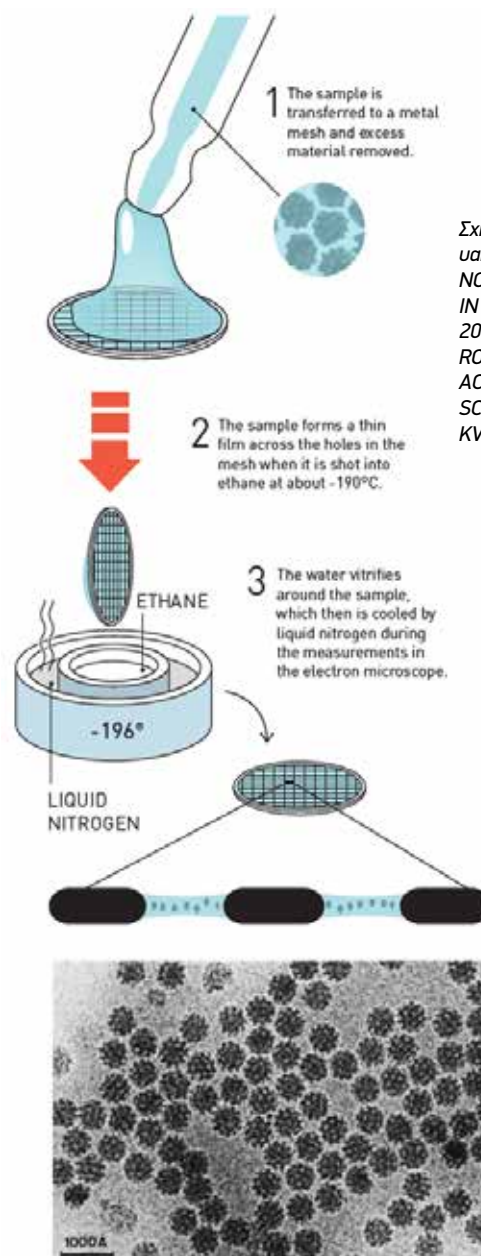
Σχήμα 1: Το Cryo-EM είναι ένα TEM (transmission electron microscope) με ειδικό χώρο δείγματος, ο οποίος επιτρέπει την παρατήρηση του παγωμένου ένυδρου δείγματος και διατηρεί θερμοκρασίες υγρού αζώτου ή υγρού ηλίου. (Royal Swedish Academy of Sciences)
